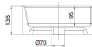
SEZIONE A-A
